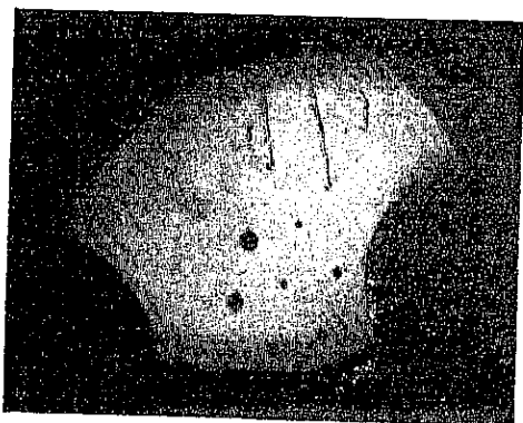
Fig. 3. Goldplatinfolie mit sieben verschieden großen Bohrungen, Einfallswinkel etwa 60^\circ .
